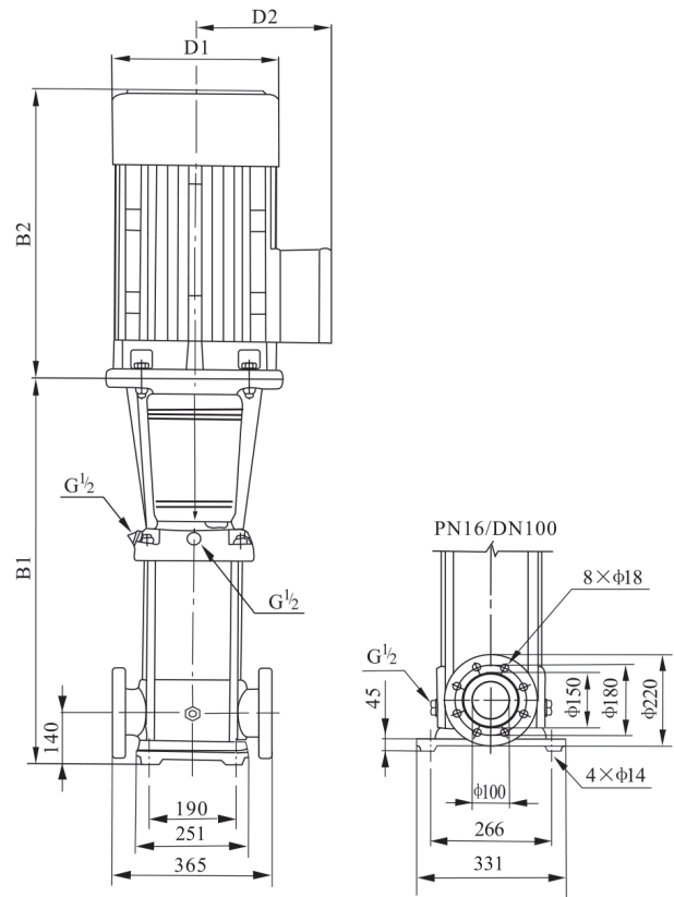
Габаритно-присоединительные размеры и вес
