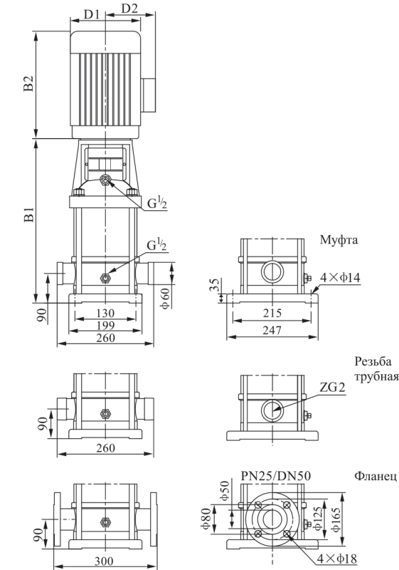
Габаритно-присоединительные размеры и вес
