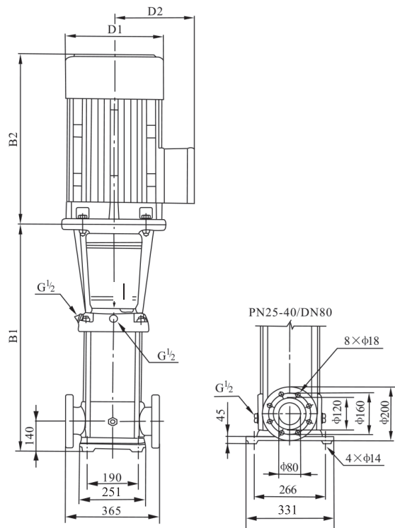
Габаритно-присоединительные размеры и вес
