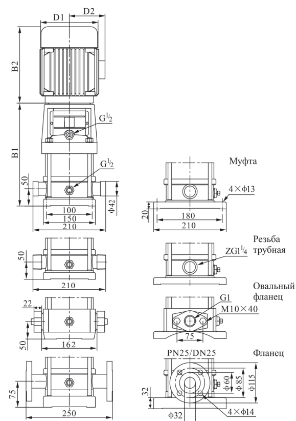
Габаритно-присоединительные размеры и вес
