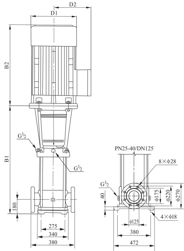
Габаритно-присоединительные размеры и вес
