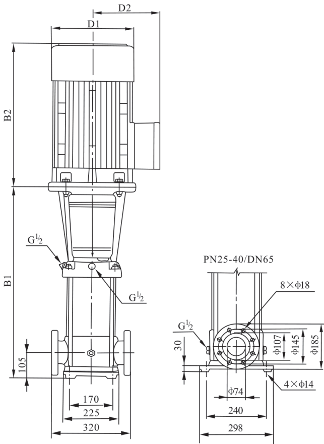
Габаритно-присоединительные размеры и вес
