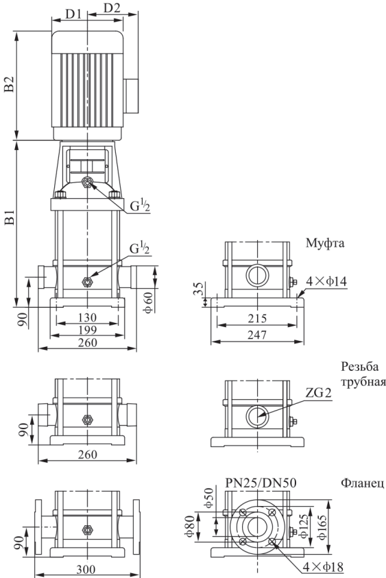
Габаритно-присоединительные размеры и вес
