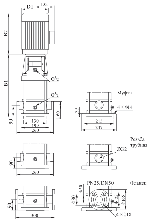
Габаритно-присоединительные размеры и вес
